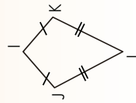
Vlieër
