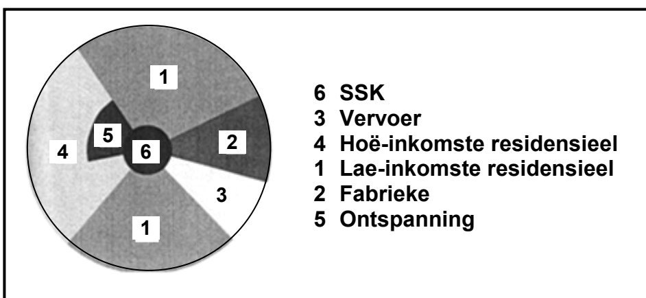
FIGUUR 3.4: GRONDGEBRUIKSONES
