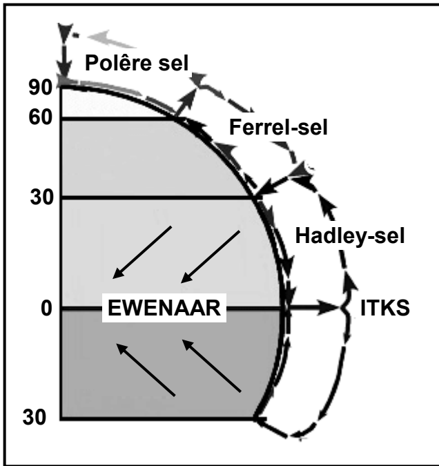
FIGUUR 1.1: DRIESELSIRKULASIE
