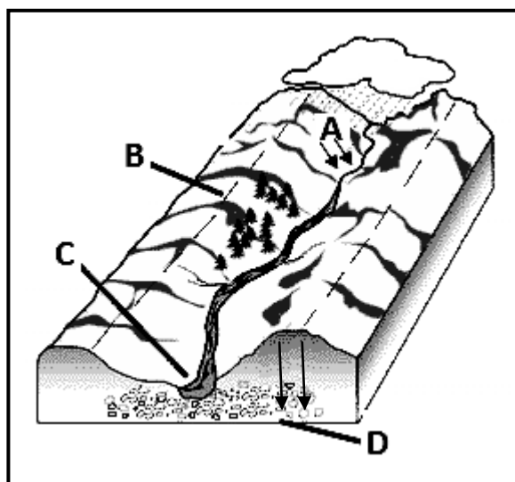
FIGUUR 2.2: RIVIERSTELSEL
