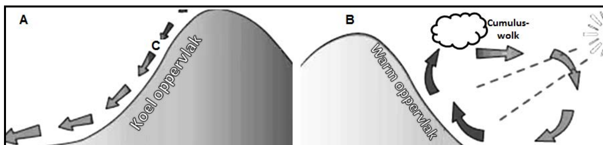
FIGUUR 2.3: PLAASLIKE WINDE
