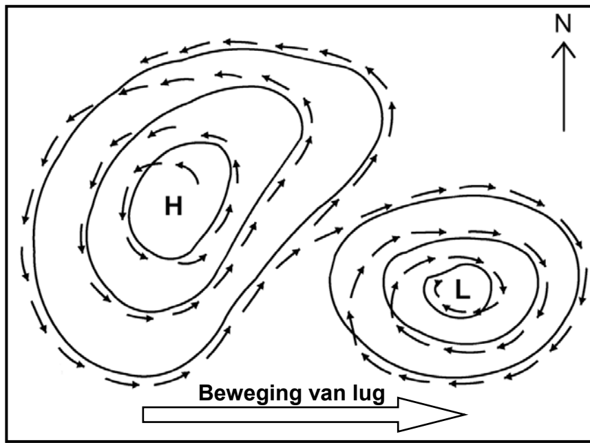
FIGUUR 2.1: HOOG- EN LAAGDRUKSELLE
