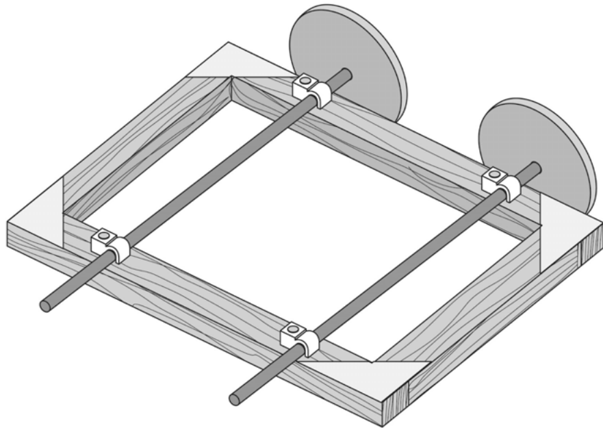
Hoe die kabelklampe die as kan vashou
