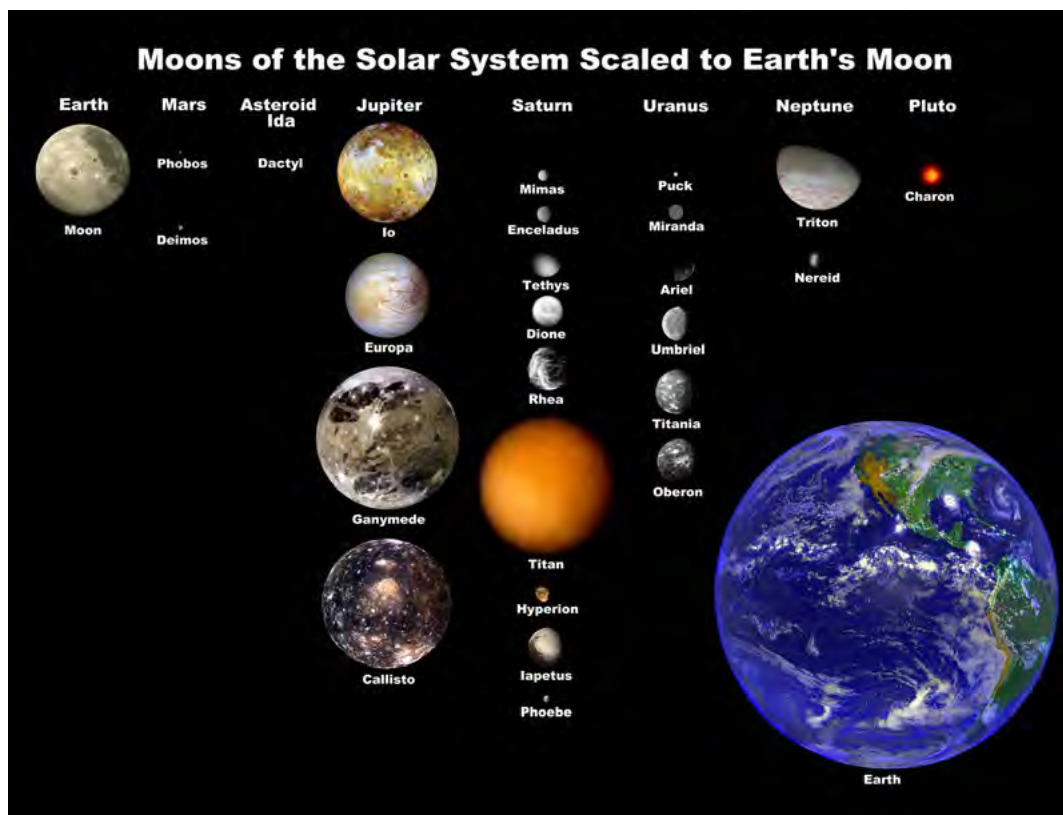
Party van die mane in ons sonnestelsel
