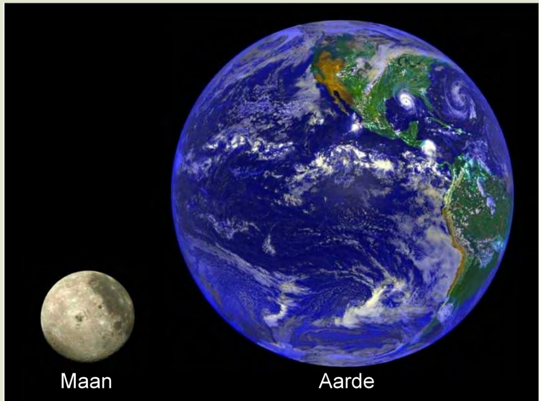
Die Maan en die Aarde - dui die verskillende groottes aan
