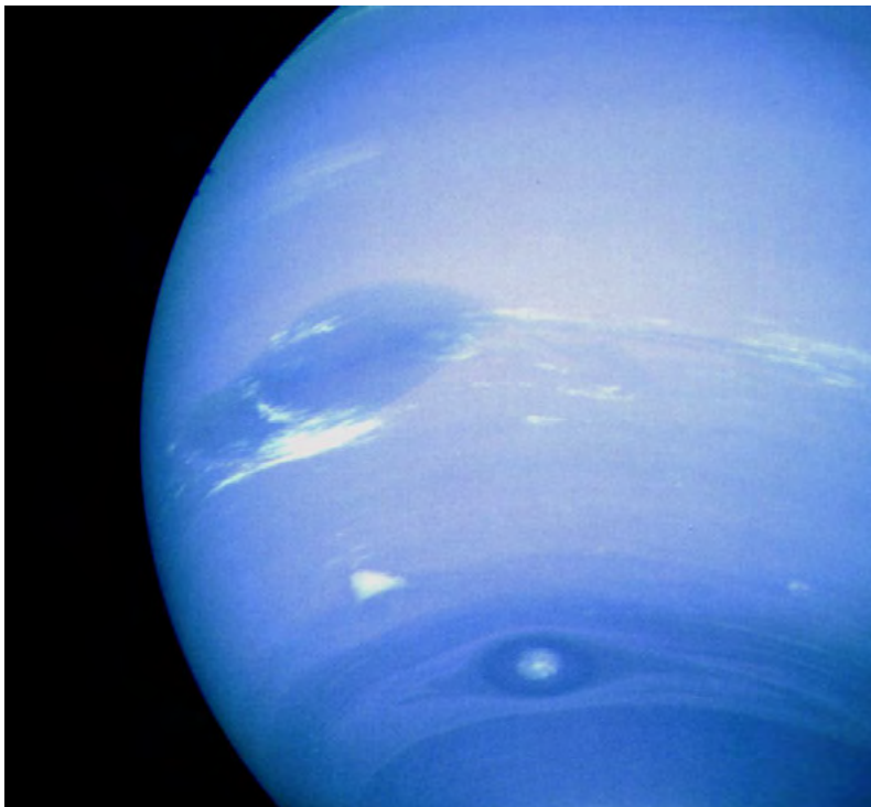
'n Naby-foto van die oppervlak van Neptunus. Kan jy die stormagtige oppervlakte sien? Dit is die donkerblou en wit kolle.
