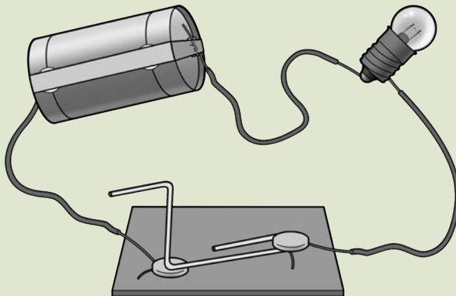
Die opstel van 'n skakelaar en 'n eenvoudige stroombaan
