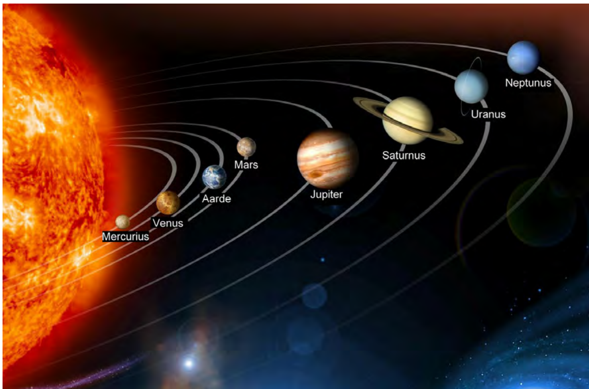
Die sonnestelsel bestaan uit die Son en 8 planete
