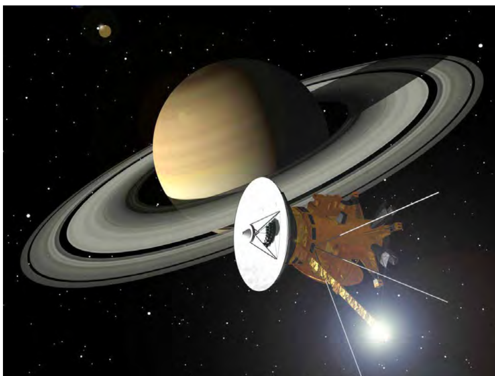
Die beeld hierbo is 'n kunstenaarsvoorstelling van die Cassini-ruimtetuig wat die planeet Saturnus en sy magnetiese ringe nader.
