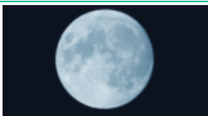
Volmaan
