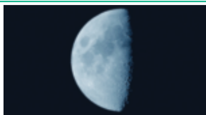
Halfmaan
