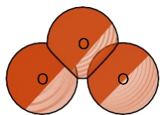
Ozone, O_3 .
